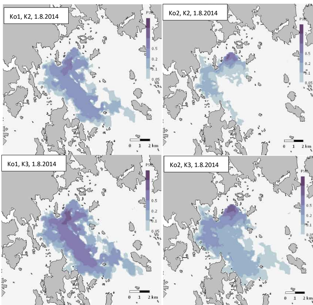
Kuva 10-30. Laskettu suolaisuuden hetkellinen pitoisuusnousu (maksimitilanne) pohjan läheisessä vesikerroksessa purkupaikkavaihtoehtoissa Ko1 (vasemmalla olevat kuvat) ja Ko2 (oikeanpuoleiset kuvat) kuormitustasoilla K2 ja K3 kesällä.
