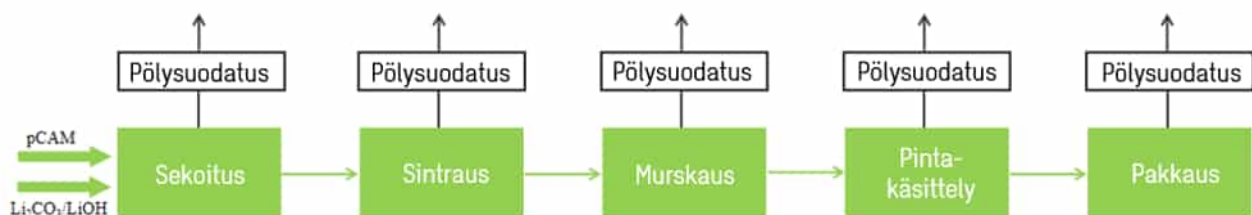
Kuva 7.1. Yksinkertaistettu CAM-tuotantoprosessi
