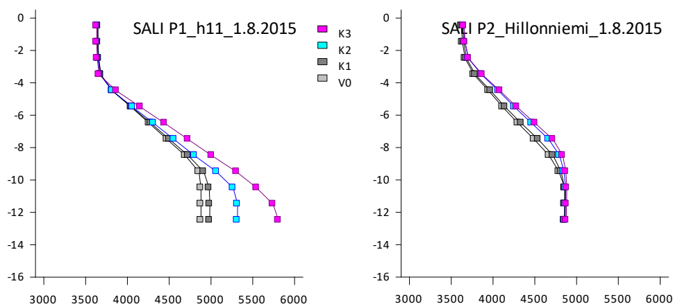
Kuva 10-38. Suolapitoisuuden (mg/l) muutos syvyyden suhteen 1.8.2014 (hetkellinen maksimitilanne) aikasarjapisteillä h11 purkupaikkavaihtoehdossa Ha1 (vasen kuva) ja pisteellä Hillonniemi purkupaikkavaihtoehdossa Ha2 (oikea kuva). V0 kuvaa nykytilaa, K1-K3 kuvaavat eri kuormitustasoja.
