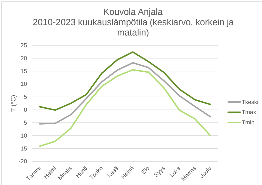
Kuva 6-7. Lämpötilan kuukausikeskiarvojen vaihtelu Kouvolan Anjalan sääasemalla vuosina 2010-2023.
