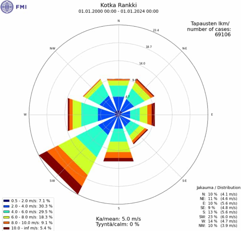
Kuva 6-8. Tuuliruusu Kotkan Rankin havaintoasemalta mitattuna vuosina 2000-2023
