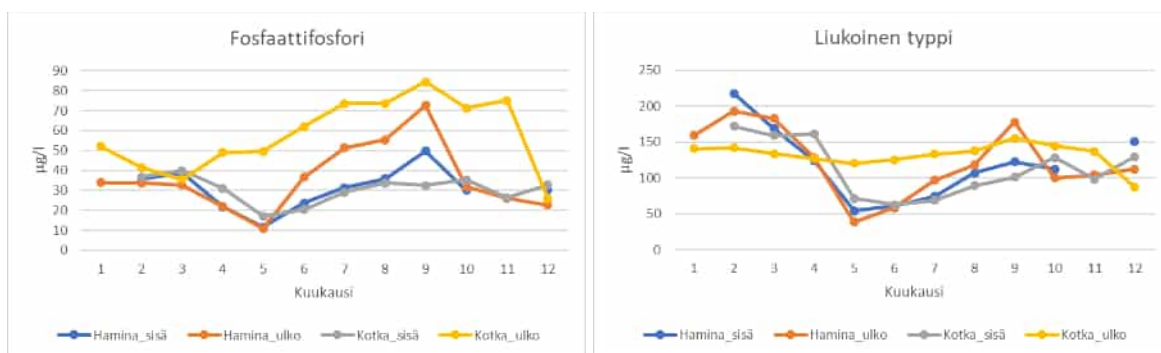
Kuva 10-21. Meriveden keskimääräinen liukoisin fosfaattifosforin ja liukoisin typen pitoisuus alusvedessä kuukausikeskiarvoina vuosilta 2010-2020.
