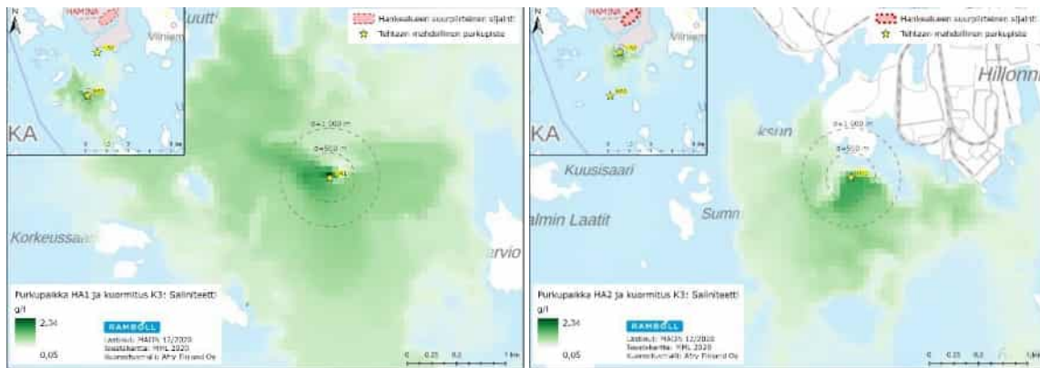
Kuva 10-39. Suolaisuuden leviäminen purkupaikkavaihtoehdossa Ha1 ja Ha2 kuormitustasolla K3. Kuviin on lisätty vyöhyke (n 500 m), jossa vaihtoehdossa Ha1 kerrostuneisuus voi olla hieman nykyistä intensiivisempää kesäaikana.
