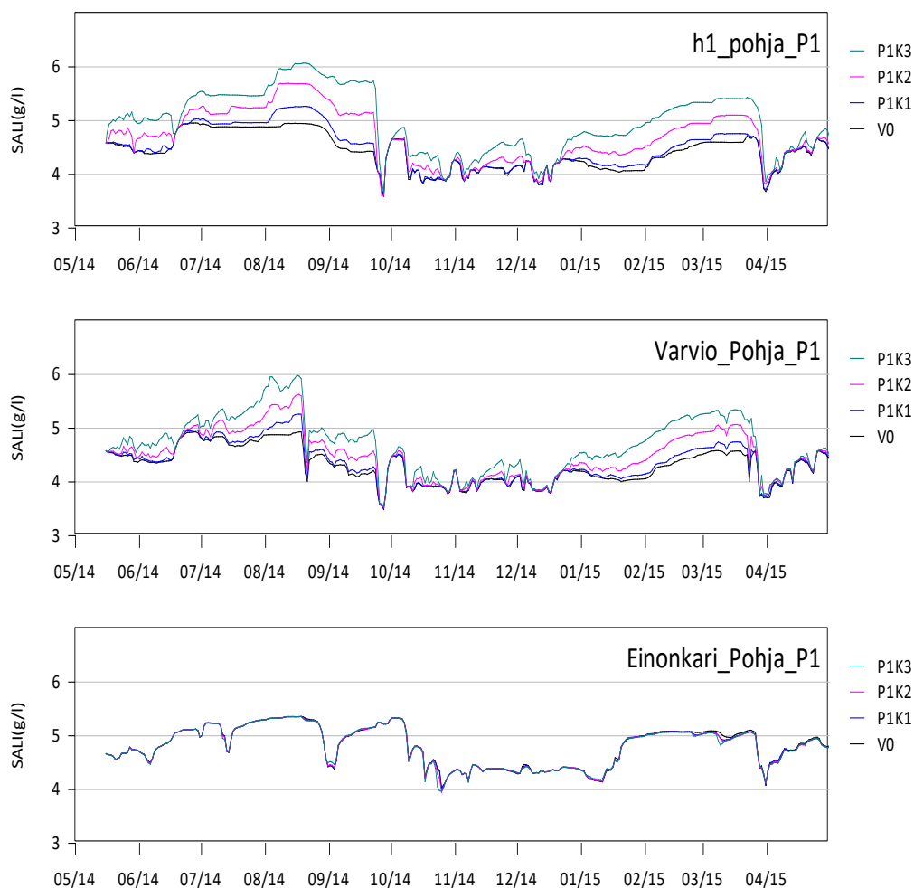
Kuva 10-35. Suolaisuuden muutokset suhteessa nykytilaan purkupisteen Ha1 läheisellä aikasarjapisteellä h1 sekä hieman kauempana pisteissä Varvio ja Einonkari. V0 kuvaa nykytilaa, K1-K3 kuvaavat eri kuormitustasoja.
