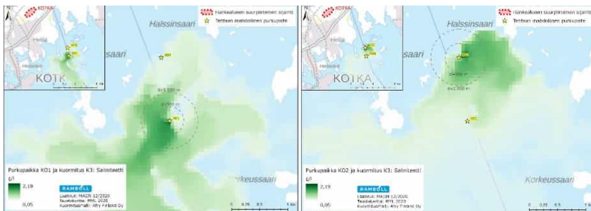
Kuva 10-32. Suolaisuuden leviäminen purkupaikkavaihtoehdoissa Ko1 ja Ko2 kuormitustasolla K3. Kuviin on lisetty vyöhyke (n. 0-1 km), jossa kerrostuneisuus voi olla hieman nykyistä intensiivisempää kesäaikana.
