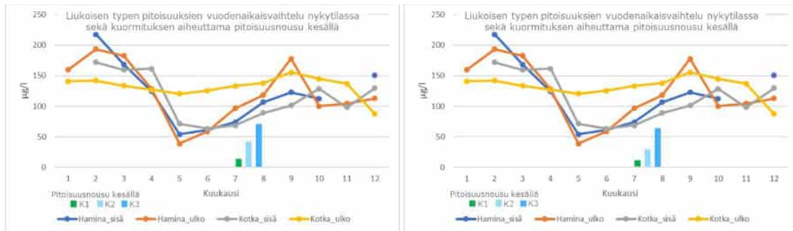
Kuva 10-41. Liukoisien typpipitoisuuden (ammoniumtyyppi ja nitraatti-nitriittitypen summa) vuotuinen kehitys sekä akkumateriaalitehtaan kuormituksesta aiheutuva pitoisuuslisäys keskikesällä (kuukausikeskiarvo) purkupaikkavaihtoehdon Ha1 lähellä (vasen kuva) ja vaihtoehdon Ha2 lähellä (oikea kuva) alusvedessä.
