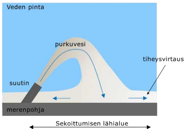
Kuva 10-5. Esimerkkikuva ympäröivää vettä tiheämmän käsitellyn prosessijäteveden sekoittumisesta yhden diffuusorin suuttimen osalta sivusta katsottuna (Jenkins ym. 2012 mukaan).
