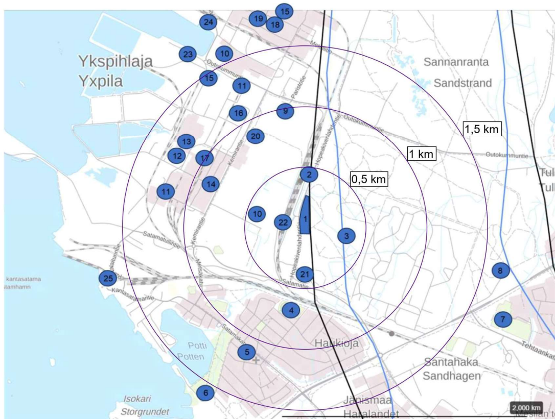
Kuva 1. LNG terminaalin ympäristö, n. 2 km säteellä. Taustakartta: kartta.paikkatietoikkuna.fi/ . Data: kartta.paikkatietoikkuna.fi/ ja kip.fi/
