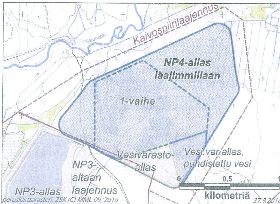
Kuva 2-5. Uuden NP4-rikastushiekka-altaan sijainti nykyisen kaivospiirin ulkopuolella (Pöyry 2016). NP4-altaan yhteyteen rakennetaan kaksi vesivarastoallasta. Uljoin vihreä viiva osoittaa patopenkereiden ulointa reunaa.
