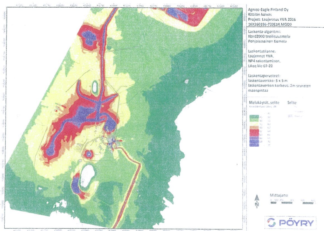
Kuva 5-6. Melun leviäminen tuotannon laajentuessa ja NP4-rikastushiekka-altaan rakennustöiden aikana, keskiäänitaso LAeq klo 07-22 (Pöyry 2016).
