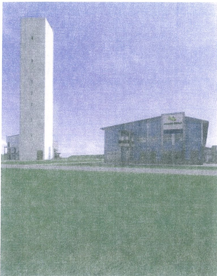
Kuva 2-2. Suunnittelun nostokuilun ja nostotornin (kuvassa vasemmalla) sijainti uuden kaivoskonttorin läheisyydessä (Pöyry 2016). Nostotornin korkeus on noin 93 metriä.
