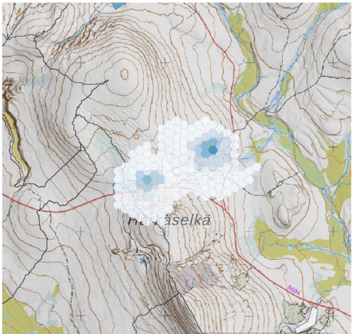
Melumallinnus härkäselän alueella Värin tummetussa ääni kovenee, solun sivun pituus on 100 m. Kartalla on esitetty 40 dB:n raja.
