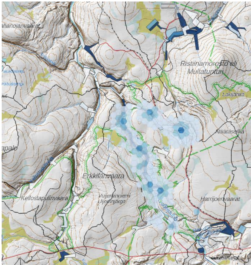
Melumallinnus Sotajoen alueella (Kutturantien ja Ivalojoen välinen alue). Värin tummetessa ääni kovenee, solun sivun pituus on 200 m. Kartalla on esitetty 50 dB:n raja.
