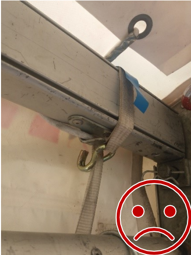
Spännbandet skärs av när det spänns.
