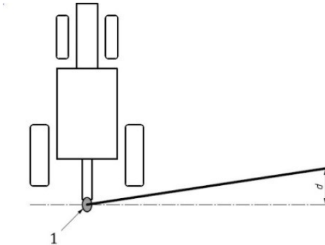
KUVA 14. Puomin virallinen enimmäisvääntymä ( d = 2,5 % puominleveydestä).
