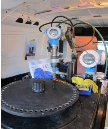
BILD 19. Testanordning för munstycken.
