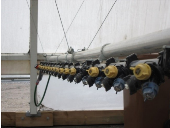
BILD 15. Från sidan ser man enkelt om munstyckena är raka.
