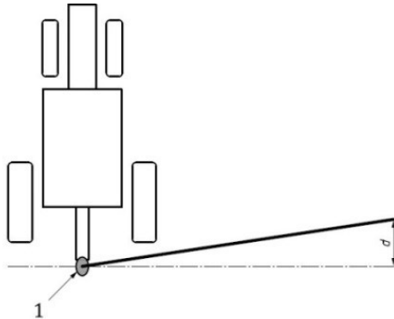
BILD 14. Den tillåtna maximideformationen av en bom ( d = 2,5\% av bommens bredd).
