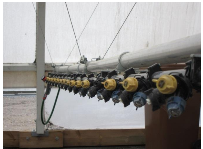
KUVA 15. Suuttimien suoruuden näkee helposti sivusta katsottuna.
