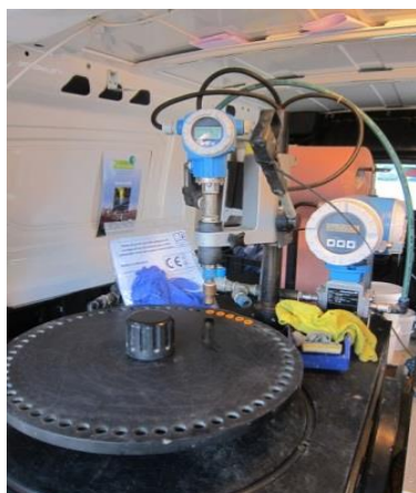
KUVA 19. Suuttimien testauslaite.
