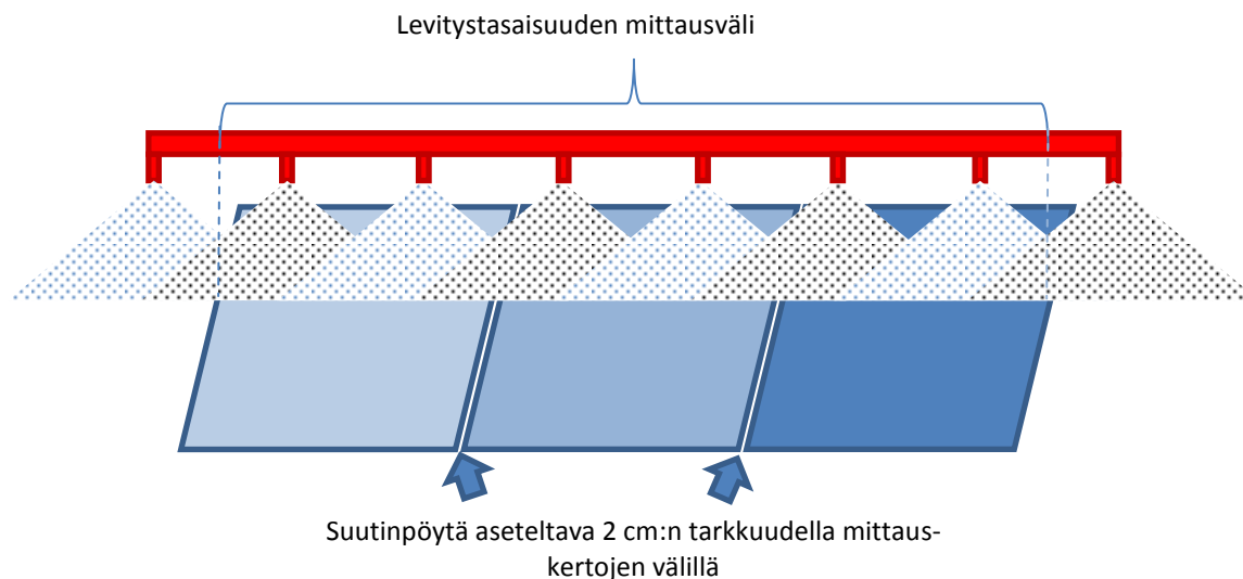
KUVA 20: Suutinpöytä tulee asettaa suutINVALMISTAJAN ilmoittamalle korkeudelle, ettei testitulostulo vääristy. Mittauskertojen etäisyys toisistaan saa vaihdella \pm 20 mm.
