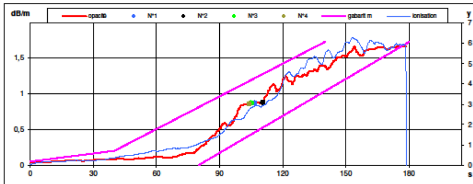
Ote testiraportista: testipalo TF4 (polyuretaani)
